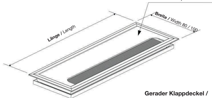
Abgerundeter Klappdeckel / Cut-Out flap Cover
