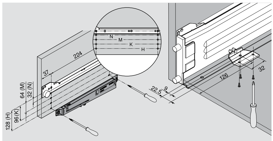
System 32: Die Montage der BLUMOTION-Einheit erfolgt im 32-mm-Bohraster.
