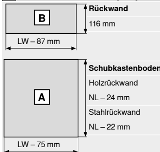
Innenschubkasten
