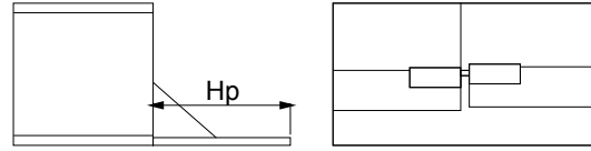
Scharnier 1 Bolzen
