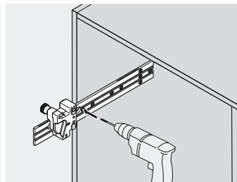
Lehre auf Riss anlegen, bohren (Ø 5 mm)
