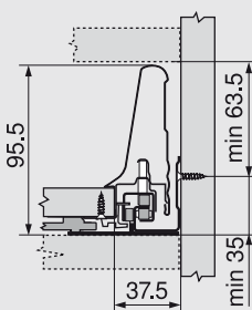
FA Frontaufschlag
