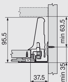
FA Frontaufschlag
