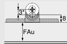
Kreuzadapterplatte
