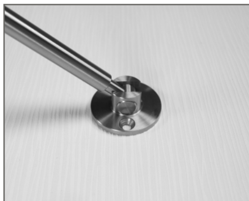
Gelenkanbindung außen (Winkel bis 90°) Rosette: Ø 45 x 3 mm (bis 5-er Spax) Gesamthöhe: 19 mm
