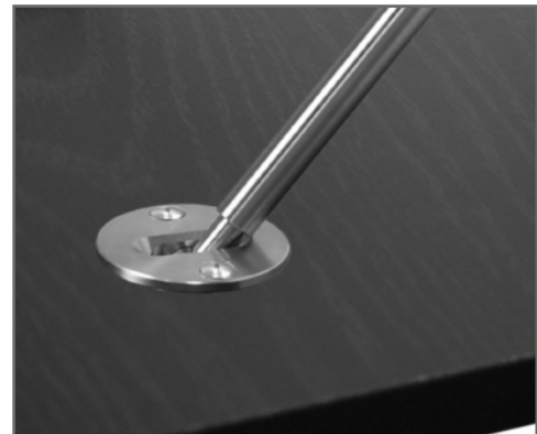
Gelenkanbindung innen (Winkel bis 45°) Rosette: Ø 50 x 3 mm (bis 5-er Spax) Bohrung: Ø 25 x 11 mm
