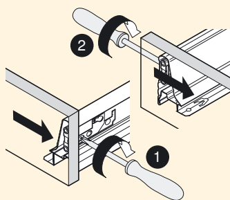
Einfach und durchschaubar, werkseitige Nulleinstellung – Justierung bei Bedarf
