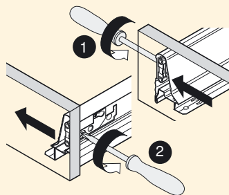
Seitliche Verstellung der Front
