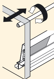
Neigungsverstellung der Front
